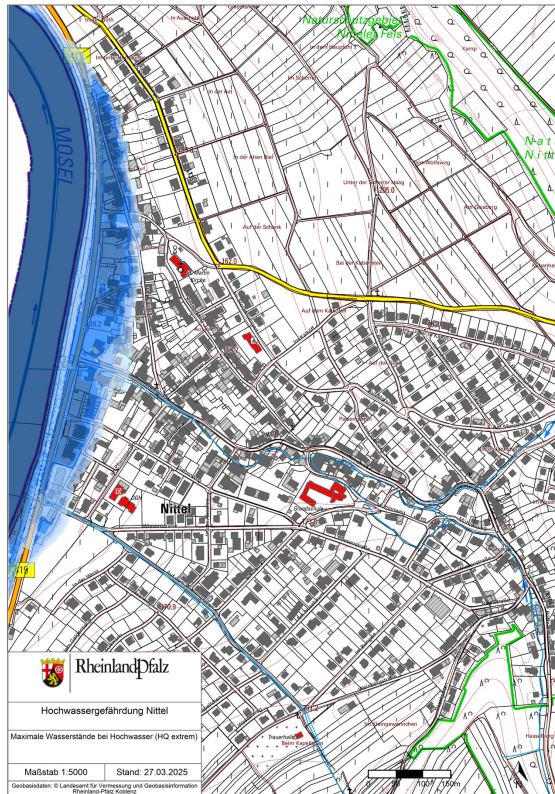
Auszug Hochwassergefahrenkarte (Nittel) mit max. Wassertiefen bei einem simulierten extremen Hochwasserereignis (HQextrem)
